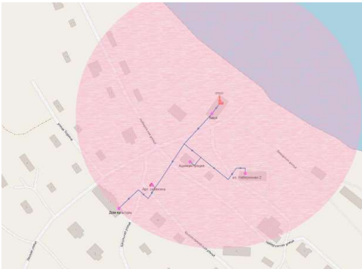
Рис. 7.15.1 – Радиус эффективного теплоснабжения котельной №1, R=175\text{м}
