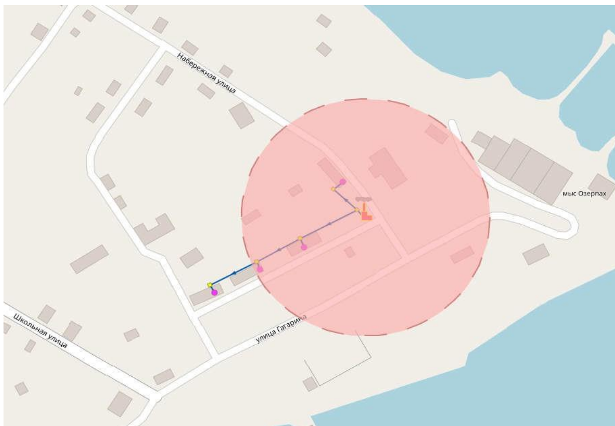
Рис. 7.15.1 – Радиус эффективного теплоснабжения котельной п. Озерпах
