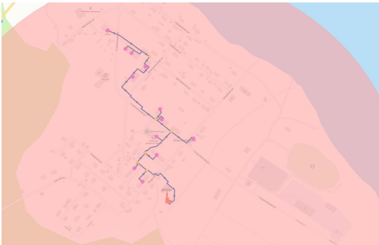
Рис. 2.5.1 – Радиус эффективного теплоснабжения котельной №1, R=811м
